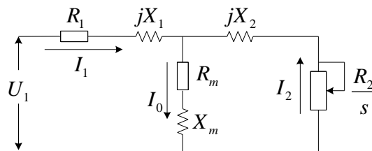
Рис. 6-12 Эквивалентная схема асинхронного двигателя
