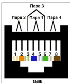
Рис. 3-15 Стандартный T568B
